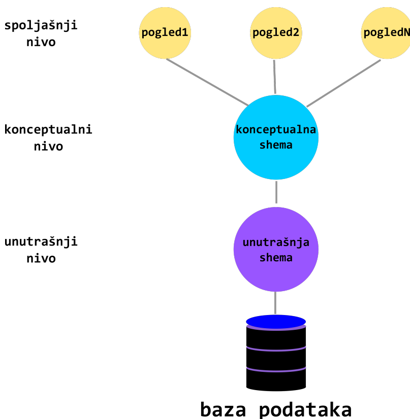
Slika 3.1: ANSI/SPARC arhitektura baza podataka
